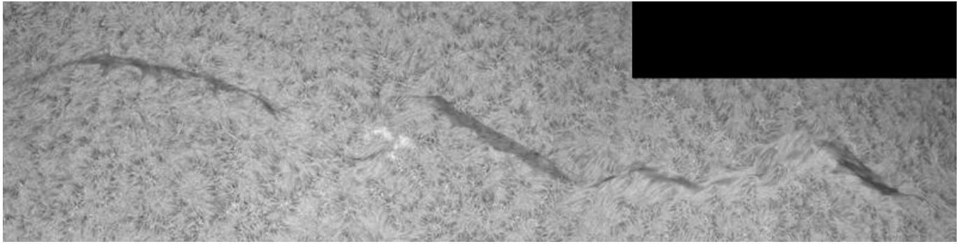
Das Bild (Mosaik) oben zeigt 3 alte Filamente, die sich bereits annähernd in Sonnenrotationsrichtung ausgerichtet haben. Solar Spectrum 0.5 Å Filter und 6" Refraktor, abgeblendet auf 90 Millimeter.
