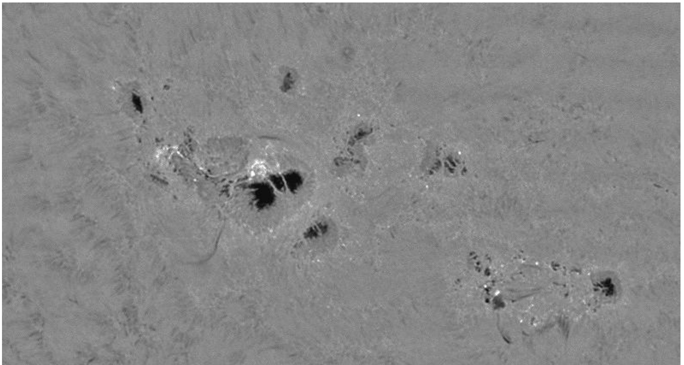
Das Bild oben zeigt Ellerman Bombs in zwei bipolaren Sonnenfleckengruppen (AR 1519 + 1520) am 10. Juli 2012. Solar Spectrum Filter während der Aufheizphase am auf 90mm abgeblendetem 6 Zoll Refraktor.
