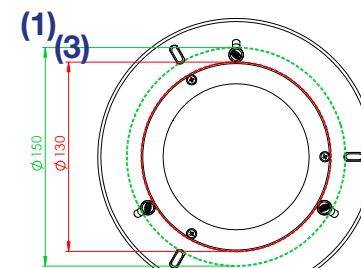
Beispiel: ASTF 100 mit 10mm Stiften
