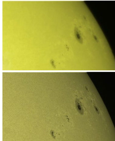
Sonne im Zeiss AS 150/2250 Refraktor bei vergleichbaren Belichtungszeiten. Oben: Herschelkeil, ND3 und ND0,9; unten: Herschelkeil, ND3 und Solar Continuum 7,5nm.
