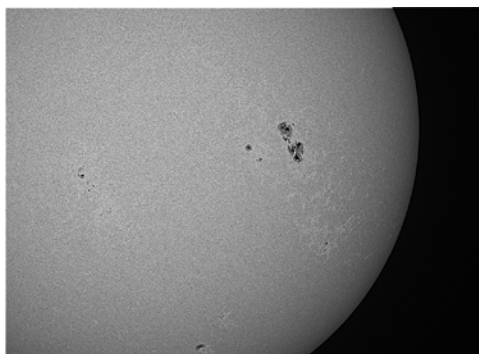
Die Sonne im Kalzium-Licht. Monochrome Kamera an Celestron ED80/600 mit Herschelkeil, ND1,8-Filter und Baader Kalzium-Filter #2961590
